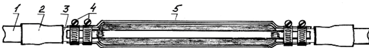
Рис. 8. Восстановление проводимости и экранирующих свойств оболочки: 1 – подброневая полиэтиленовая оболочка; 2 – трубка ТУТ продольной герметизации; 3 – алюминиевая оболочка; 4 – червячные хомуты из нержавеющей стали (4 штуки); 5 – алюминиевые полосы (4 штуки).
